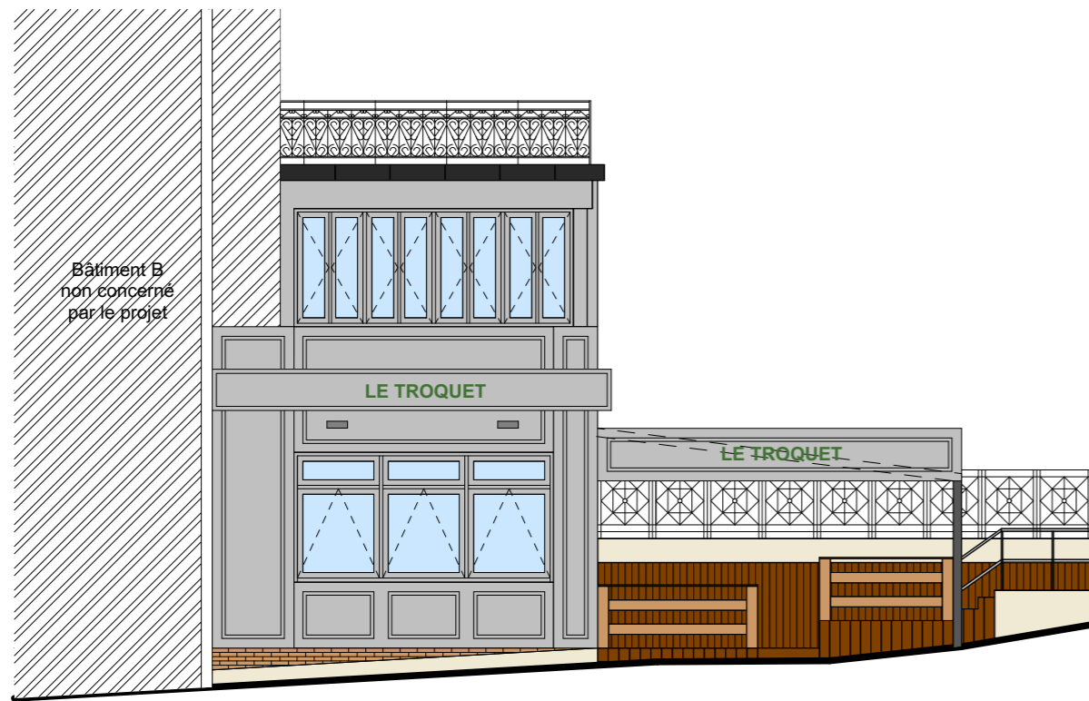
Façade Ouest (projet)
